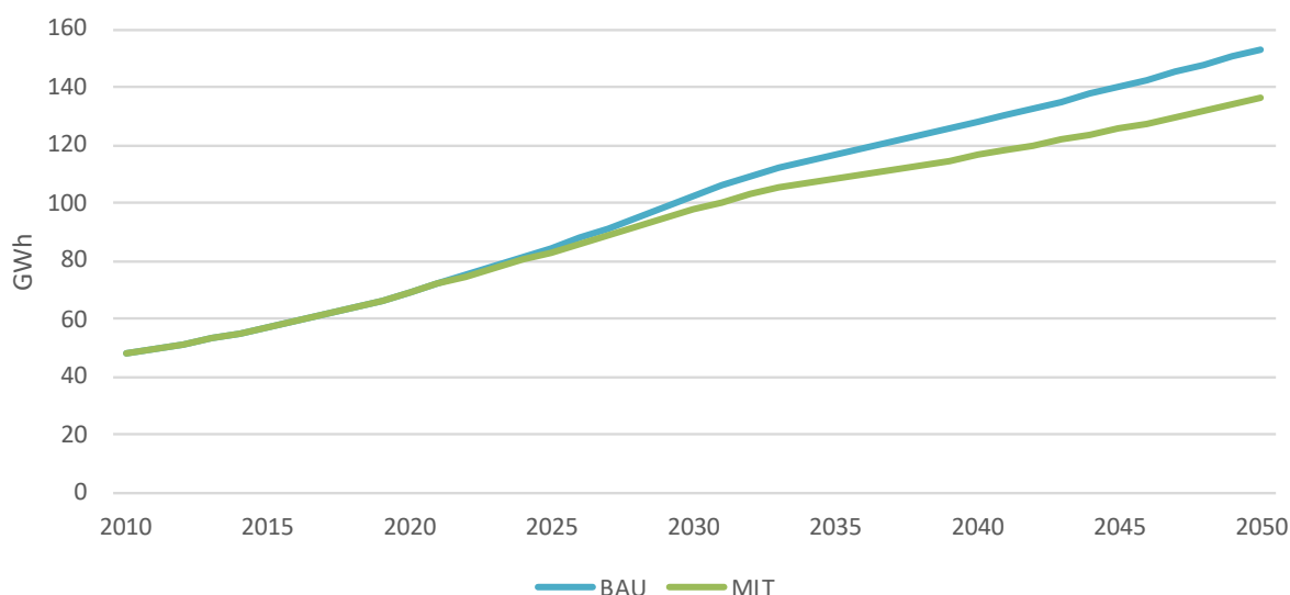
Figure 41: Consommation d'énergie prévue dans le secteur RAC industriel dans le scénario BAU et le scénario de mitigation (MIT). (Source : Analyse HEAT)
