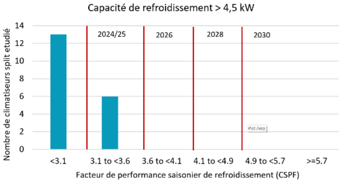
Figure 18: Distribution de fréquence de l'efficacité énergétique des CA étudiés avec une capacité de refroidissement > 4.5 kW à 9.5 kW (basée sur le CSPF estimé pour le groupe climatique 0A), les lignes rouges et les années indiquent les SMPE proposées.
