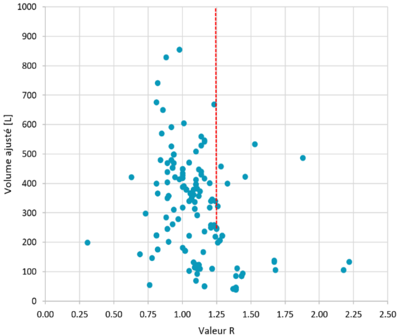
Figure 9: Relation entre le volume ajusté (AV) des réfrigérateurs étudiés et la valeur R (Source : analyse HEAT).
